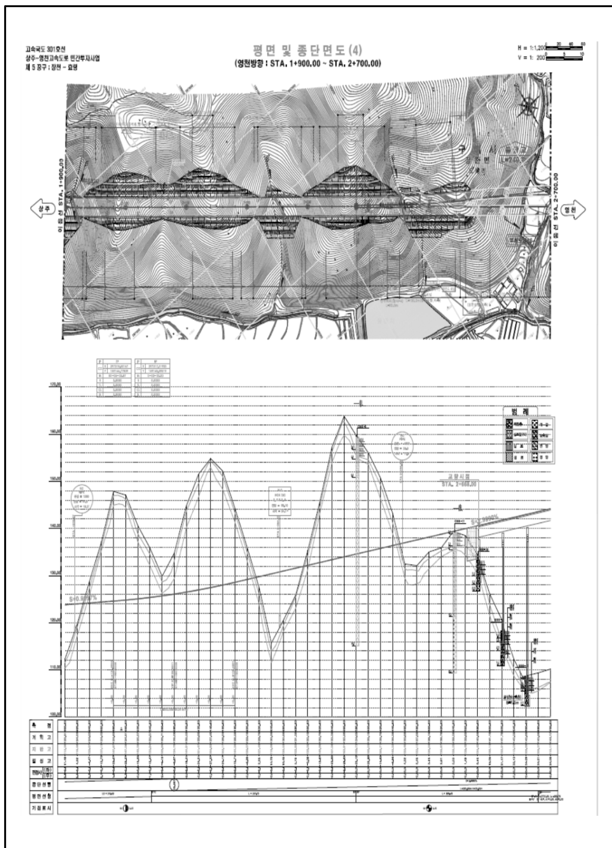
【그림 29.3】 평면도
