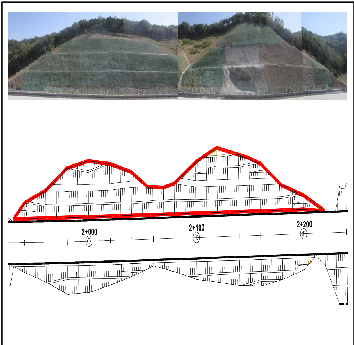
【그림 29.14】 상주절토29 검토대상 비탈면구간
